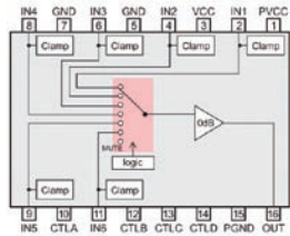
BH76362FV
